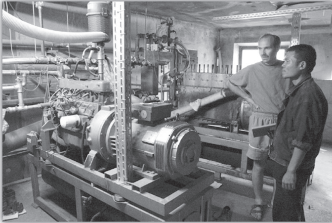
เครื่องกำเนิดไฟฟ้ารุ่นแรกของชวานา
